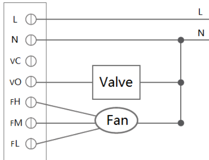
Fig. 2. Honeywell VC4013/VN4013/VS4016 Wiring
